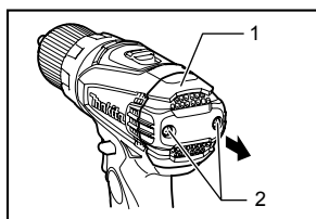
1. Couvercle arrière 2. Vis
