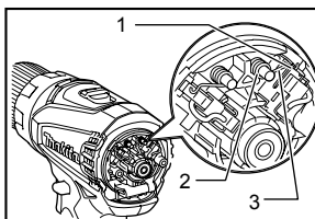
1. Partie encastrée 2. Ressort 3. Bras
